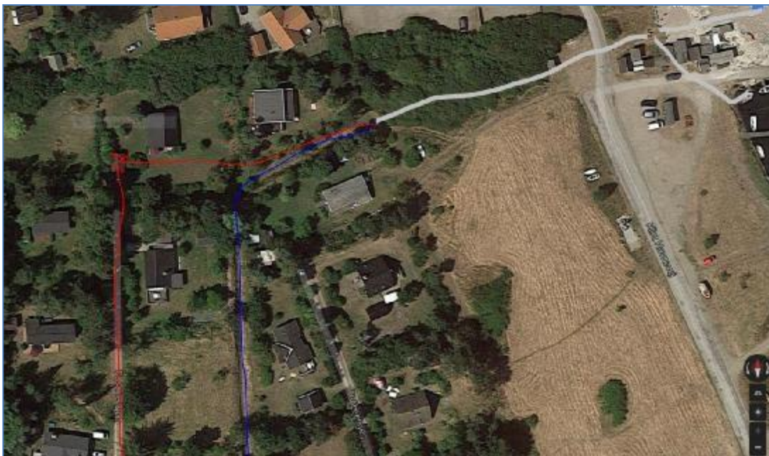
Kabelføring, strøm til pumpestation vist med rødt. Grøften vist med blå og rørlægningen med gråt.
